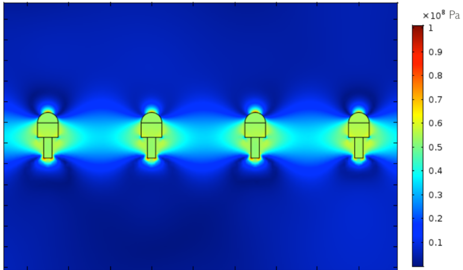
Amplitud av oscillerade spänning \sigma_{xx} vid ca 27 Hz.
