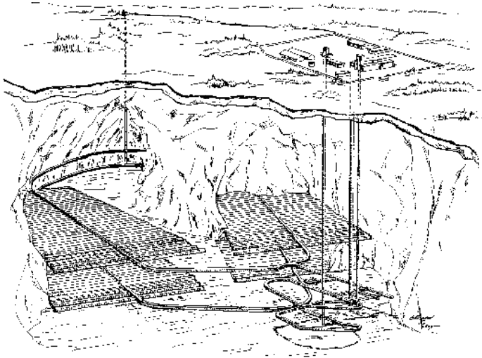
Skiss på slut för varen ligt KBS-metoden.
