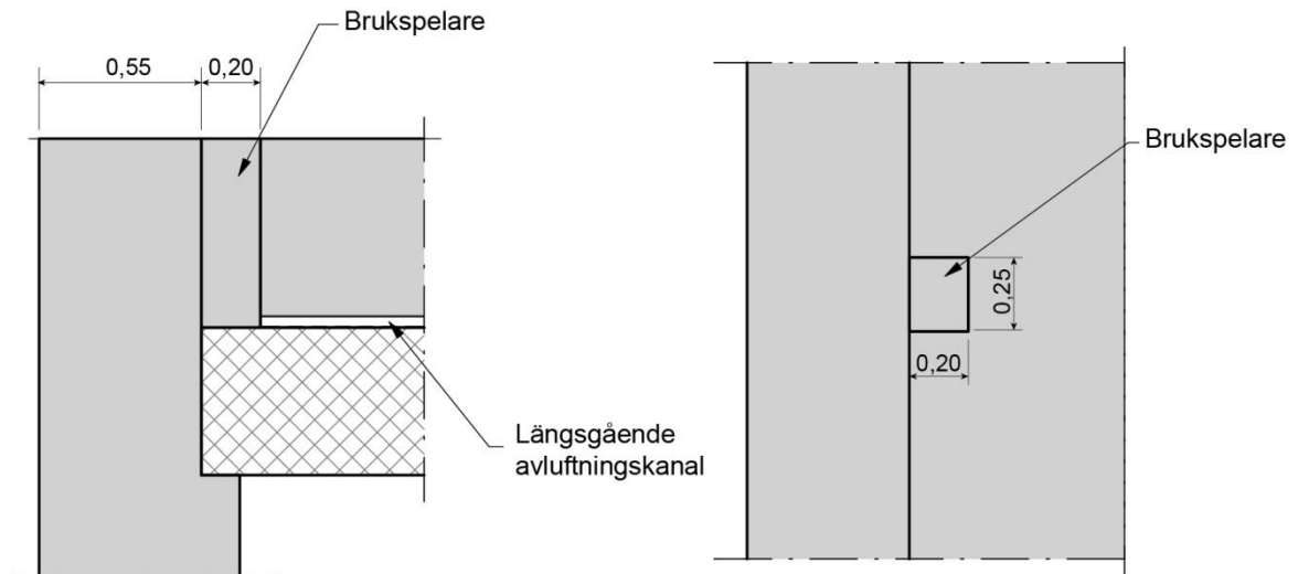
Figur 3-4. Vertikal gasavlastningskanal fylld med poröst cementbruk; genomskärning till vänster och sett från ovan till höger. Ytterväggen ses till vänster i båda figurerna och det pågjutna locket till höger. I genomskärningen (till vänster) ses även strålskärmslock (rutat). Mått i meter.
