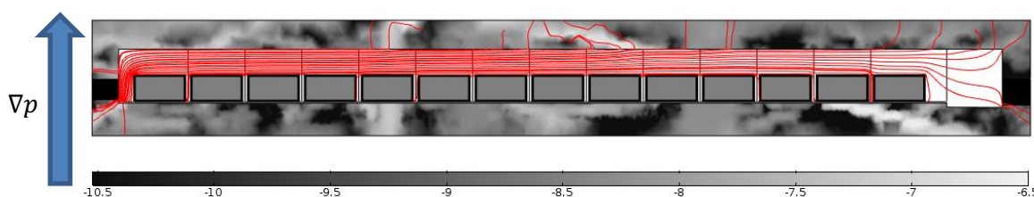
Figur 4-4. Strömlinjer som illustrerar den lokala flödesbilden vid 2000 e Kr i ett vertikalt plan som skär 2BMA. Gråskalan visar logaritmen av den hydrauliska konduktiviteten i berget, \log(K) (m/s). Den blå pilen indikerar tryckgradientens huvudkomponent i berget.
