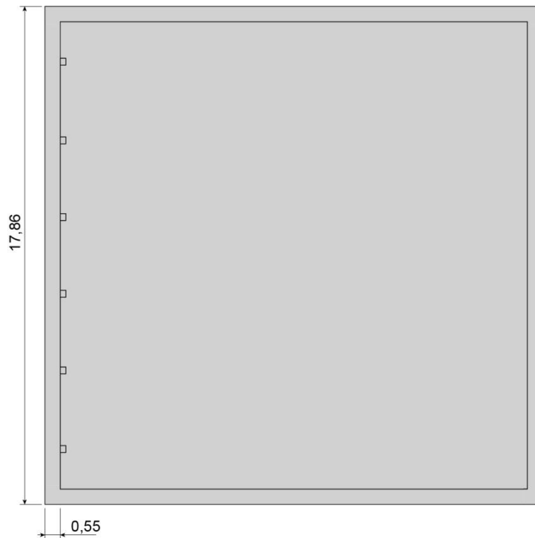
Figur 3-5. Betongkonstruktionens lock sett från ovan. De vertikala gasavlastningskanalerna med poröst cementbruk placeras längs med en yttervägg och kan ses i vänsterkanten på betongkonstruktionens lock i figuren. Mått i meter.
