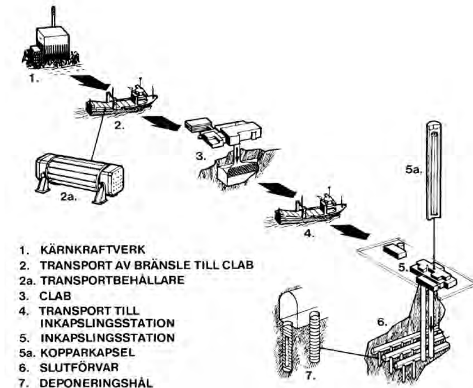
Figur B-6. Hanteringsgång för använt kärnbränsle /SKBF/KBS 1983, Del I sid 2:4/.
