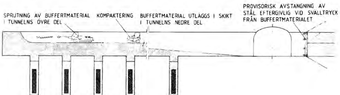
Figur B-7. Vid försegling av slutförvaret fylls tunnarna med en blandning av kvartssand och bentonit. Det undre lagret utläggs med traktorer och vibrovältas. Den övre delen av tunneln fylls genom sprutning /SKBF/KBS 1983, Del I sid 4:14/.
