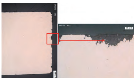
Figur 2. Omfattande kopparkorrosion och gropfrätning i FEBEX-försöket. Källa: "FEBEX-DP Metal Corrosion and Iron-Bentonite Interaction Studies, P. Wersin & F. Kober, NAB 16-16, Nagra October 2017.
